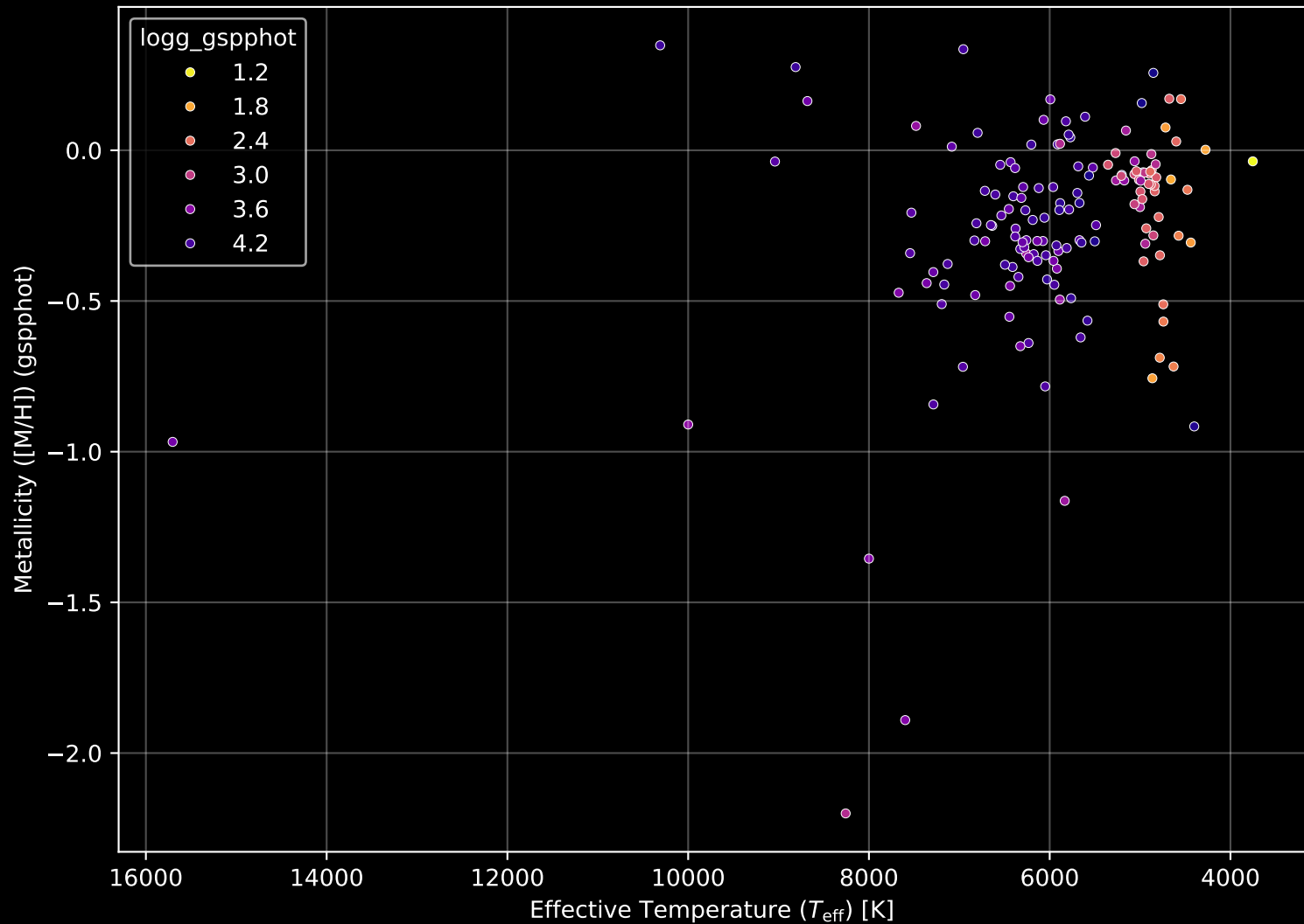
GALAH DR4 Field: [3728] Stellar Population Parameters (n= 150)
