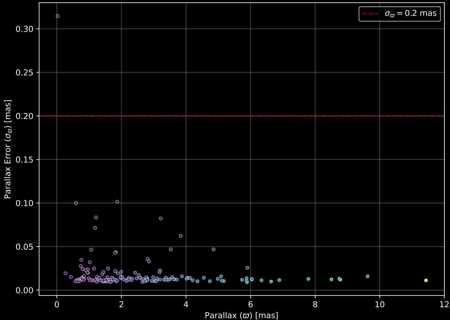
GALAH DR4 Field: [3728] Parallax Quality (n= 150)
