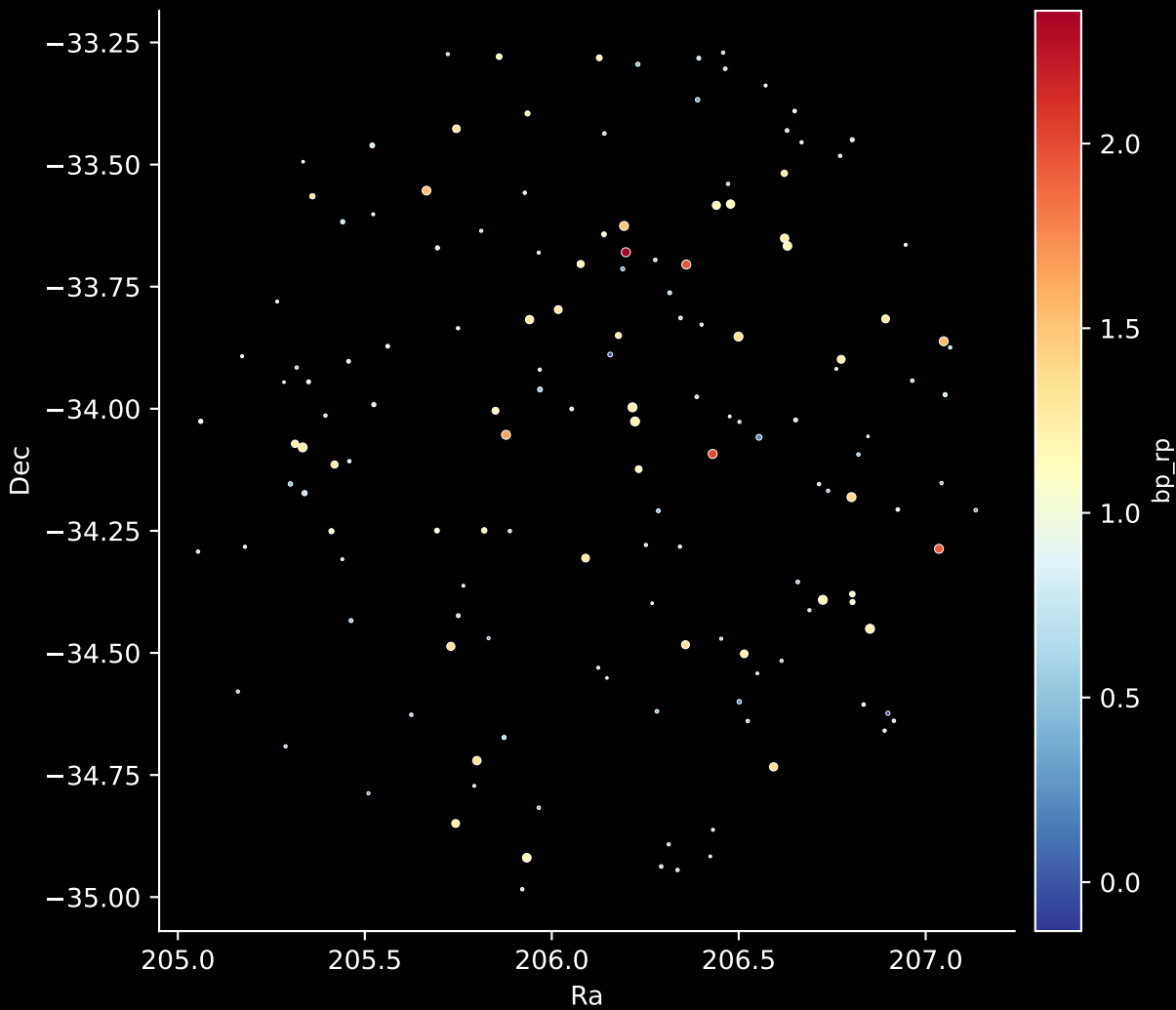
GALAH DR4 Field: [3728] Stars: 150
