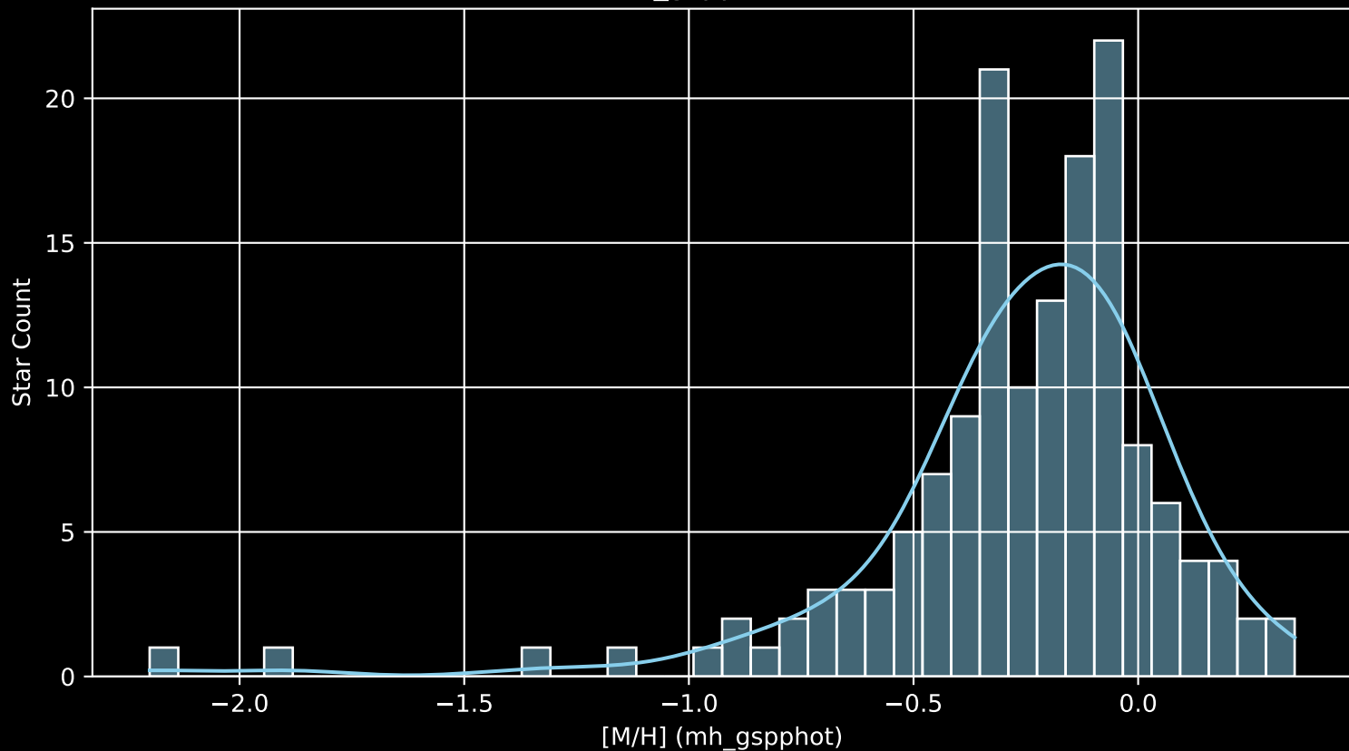
GALAH DR4 Field: [3728] [M/H] (mh_gspphot) (n= 150)
